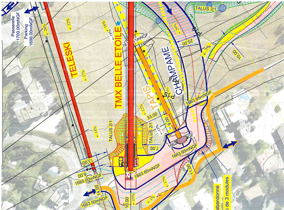
fig. 2. Extrait de la gare aval du TSCD Belle Etoile
