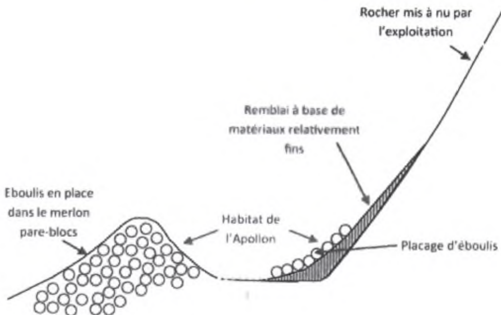
Coupe type en fin d'exploitation
