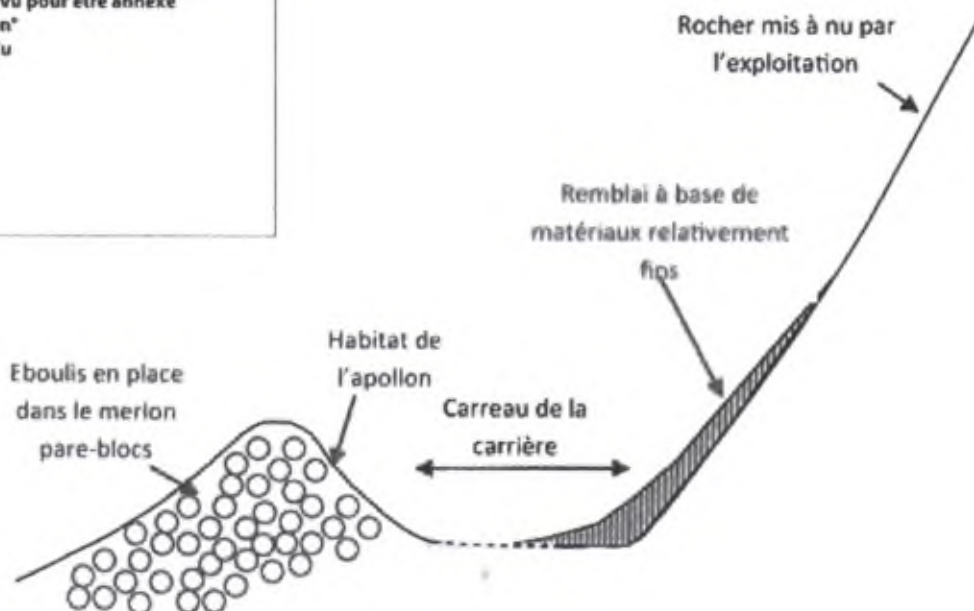
Coupe type en phase d'exploitation
